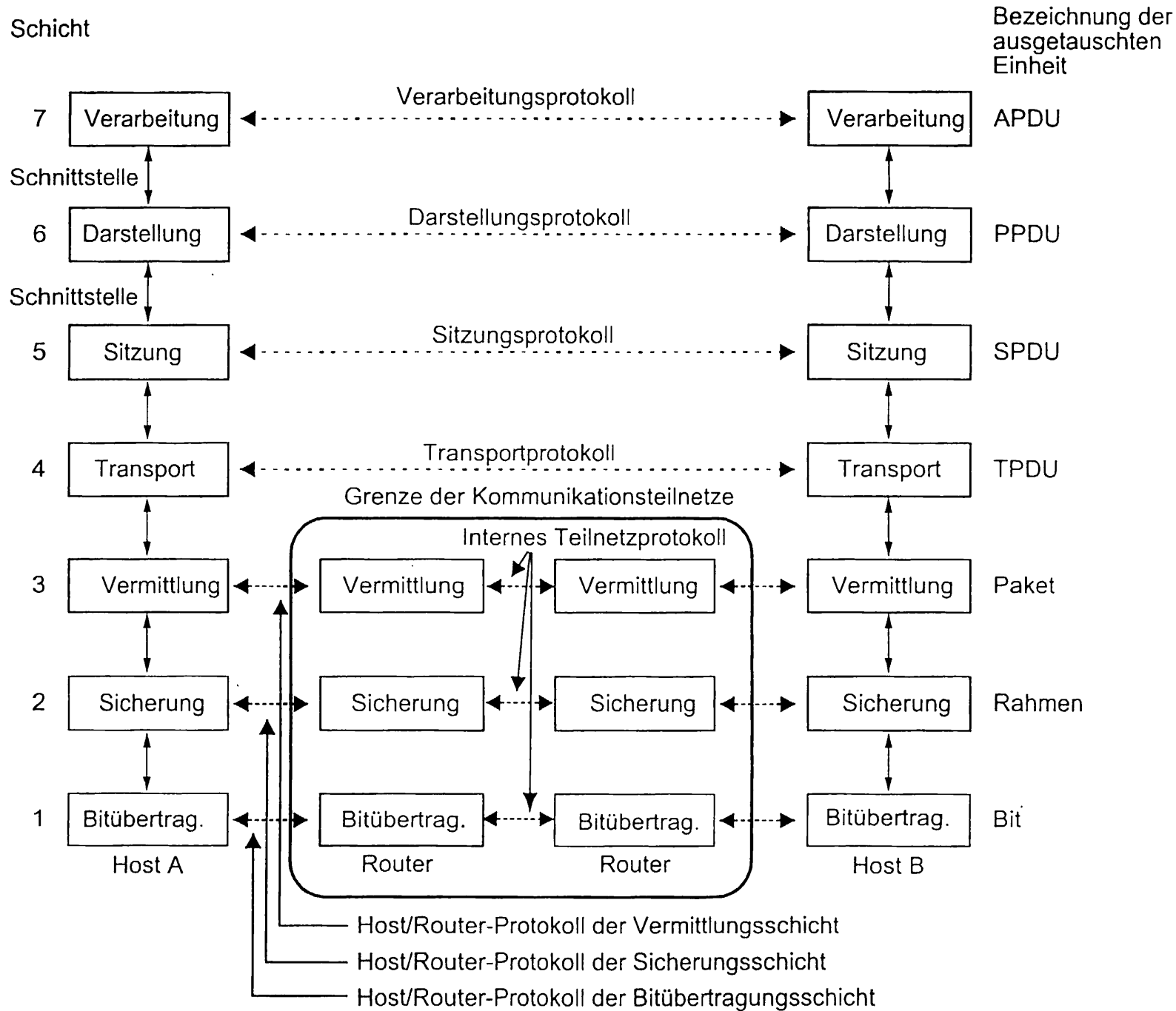
Abb. 1.16: Das OSI-Referenzmodell
